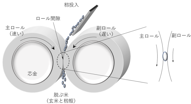
図1 ロール籾摺り機の模式図
