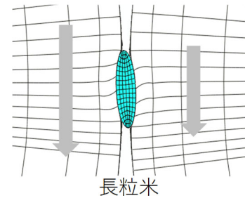
図2 ロール間隙での籾の挙動
