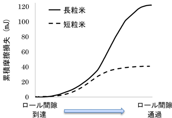
図3 籾1粒当たりの累積摩擦損失
