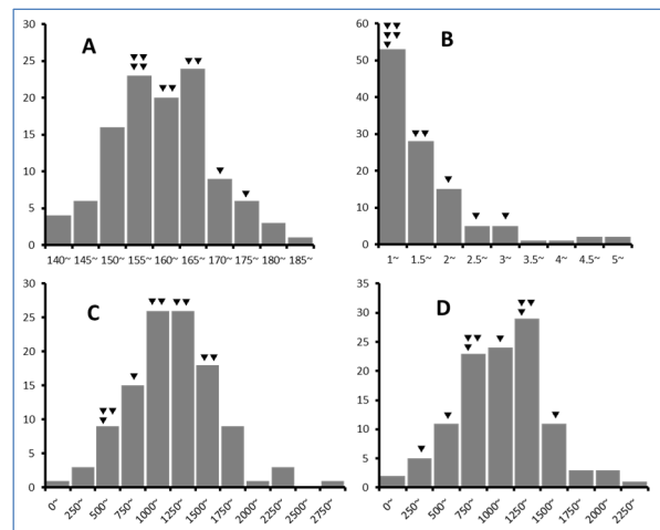
図3 DrDRS 系統の基礎農業形質における変異
