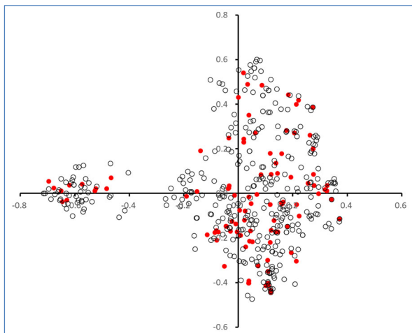
図2 SSR 多型に基づく主座標分析における元集団と DrDRS 系統の分布
