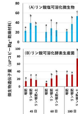
図2 堆肥化中のリン酸塩可溶性微生物量とリン酸可溶性酵素量の推移 (A)リン酸塩可溶性微生物=リン酸塩可溶性糸状菌+リン酸塩可溶性細菌、(B)リン酸可溶性酵素生産菌=アルカリホスファターゼ生産菌+酸性ホスファターゼ生産菌+ホスホナターゼ生産菌。各サンプリング期間で異なるアルファベットは一元配置の分散分析により p < 0.05 で有意差があることを示す。
