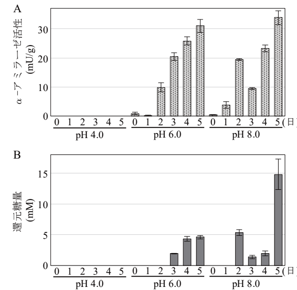
図 3 酸緩衝液 (pH 4.0, 6.0, 8.0) による浸漬処理の後、37℃で 5 日間保温した麺における α-アミラーゼ活性 (A) および還元糖量 (B) の消長
