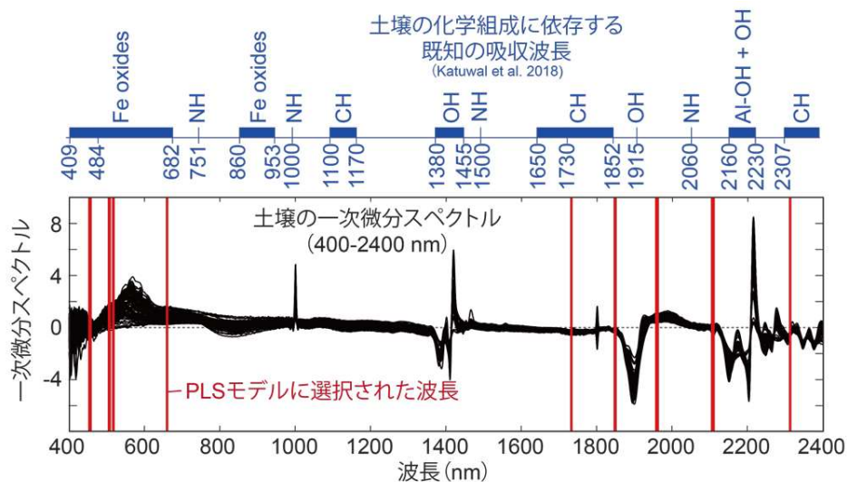
図3 PLSモデルで選択された波長
