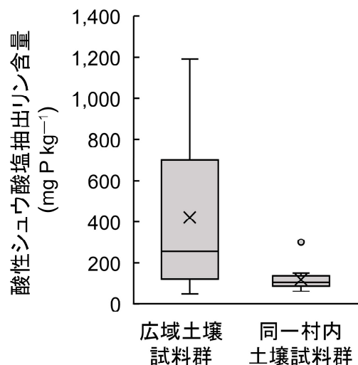
図1 酸性シュウ酸塩抽出リン含量の空間変動
