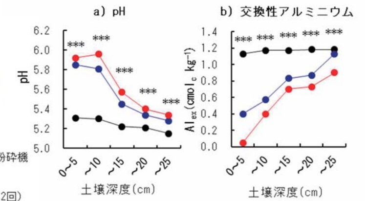
図 2 ナノ加工石灰の移動に伴う土壌化学成分の変化
