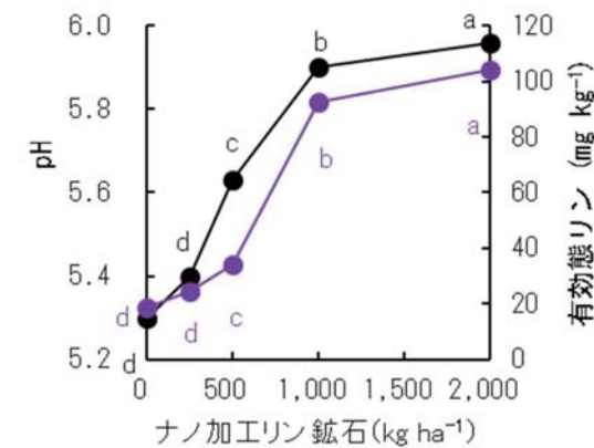
図 3 ナノ加工リン鉱石施用による土壌化学成分の変化
