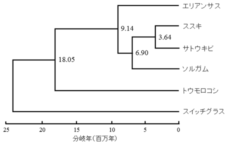
図2 葉緑体ゲノムに含まれる 76 種類のタンパク質コード領域の多様性にもとづくイネ科植物の分岐年代 図中の数値は、推定分岐年代を示す。
