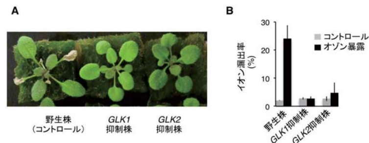
図 1. GLK1, GLK2 転写因子の機能を抑制した植物のオゾン耐性 A, 0.3 ppm のオゾンに 7 時間処理後一日目の植物の様子。 B, オゾン処理後植物 (第 2 葉) の障害の程度の評価。グラフは 3 反復の平均値 (1 反復 3 植物を使用)、エラーバーは SD 値を示す。 図は Nagatoshi Y et al. (2016) を改変 (Copyright: National Academy of Sciences, USA)。
