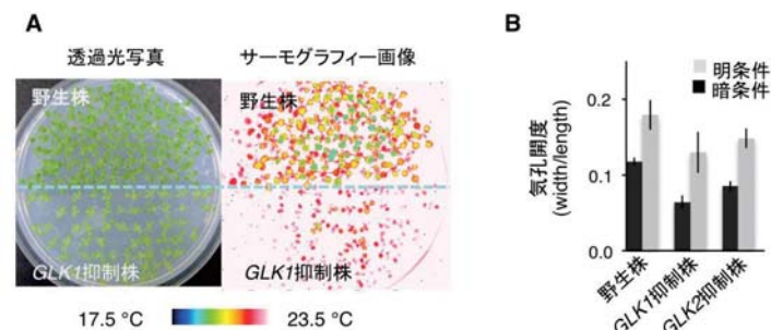
図 2. オゾン耐性を持つ GLK1, GLK2 抑制植物の気孔開度 A, 培地で 2 週間生育した植物 (左) のサーモグラフィ画像 (右)。 B, 培地で 2 週間生育した植物の気孔開度。グラフは 3 試験の平均値 (1 試験約 50 個の気孔を観察)、エラーバーは SD 値を示す。 図は Nagatoshi Y et al. (2016) を改変 (Copyright: National Academy of Sciences, USA)。
