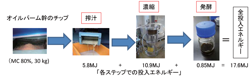
図 1 オイルパーム廃棄木からのエタノールを生産する際の搾汁、濃縮、発酵の各プロセスに要する投入エネルギー
