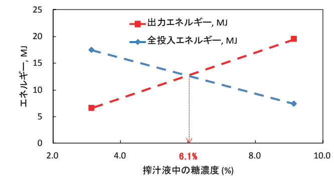
図 3 エネルギー収支がプラスに転じる搾汁液中の糖濃度
