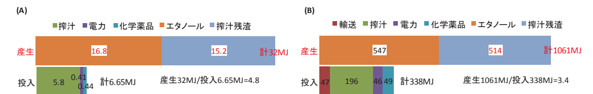
図2 搾汁に関わるエネルギー (A)トランクコア (20cm x 1.2m) (B)全トランク(40cm x 10m) 全トランクの場合はプランテーションからの輸送エネルギーが加算される
