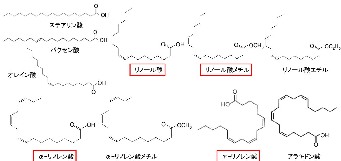
図1 各種脂肪酸および脂肪酸エステル(囲みのある物質に活性あり)
