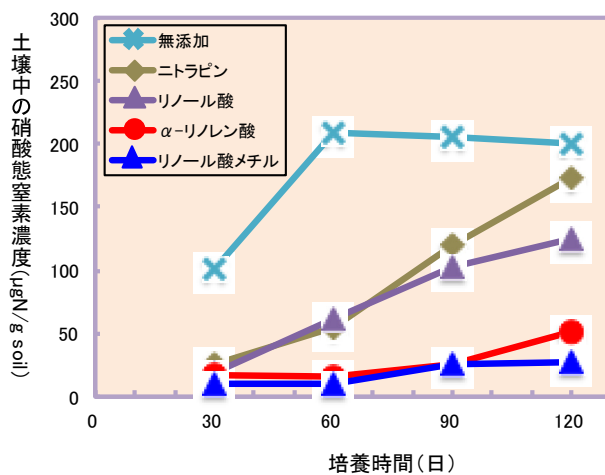
図3 各物質添加土壌での硝酸態窒素濃度の経時的変化(室内試験)
