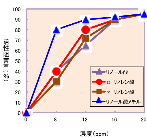
図2 各物質の濃度と硝化細菌 Nitrosomonas europaea の活性阻害との関係
