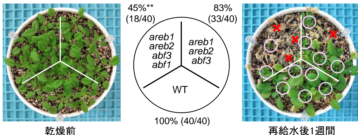
図1 AREB/ABF型転写因子の機能を欠損させたシロイヌナズナ多重変異体の乾燥ストレス耐性 4個のAREB/ABF型転写因子の機能を欠損させた areb1 areb2 abf3 abf1 四重変異体、3個のAREB/ABFの機能を欠損させた areb1 areb2 abf3 三重変異体および野生型株 (WT) シロイヌナズナの乾燥ストレス耐性試験の結果を示す。写真は、代表的な供試ポットの乾燥ストレス前後の様子を示す。GM寒天培地上で3週間生育させた植物を土植えにし、その後1週間生育させ、給水を停止することにより乾燥ストレスを与えた。乾燥ストレス開始後11-12日目に再給水を行い、1週間後に写真撮影を行った。○印と×印は、それぞれ生存個体と死滅個体を示す。1回の実験で8個のポットを用いて実験を行い、3回の反復実験を行った。中央の模式図には、代表的な1回の実験の結果をもとに計算した生存率 (生存個体数/総供試個体数) を示した。 ** P < 0.01 ( t -検定、野生型株との比較)
