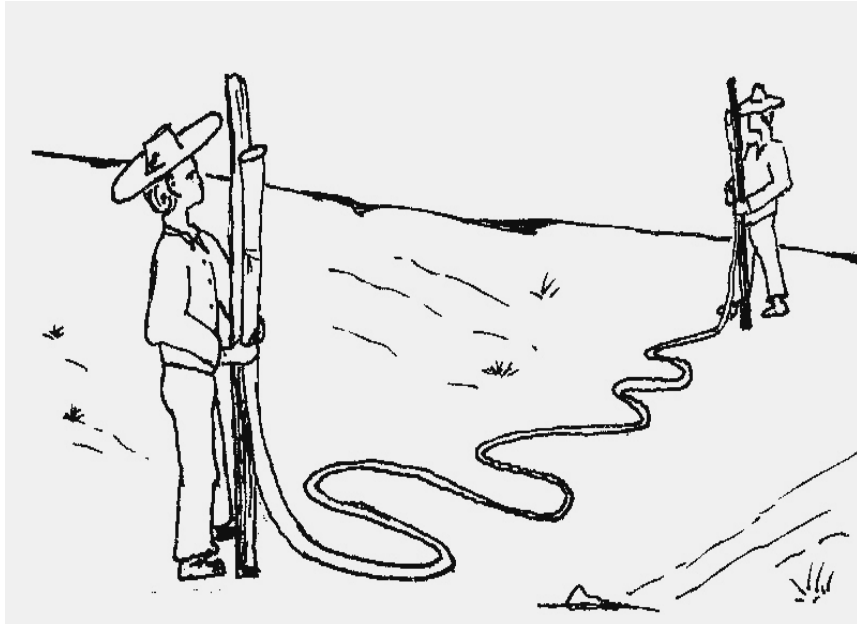
Figura 4: Calibración del nivel de manguera
