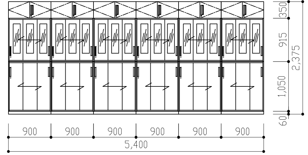
参考: 収納立面図
