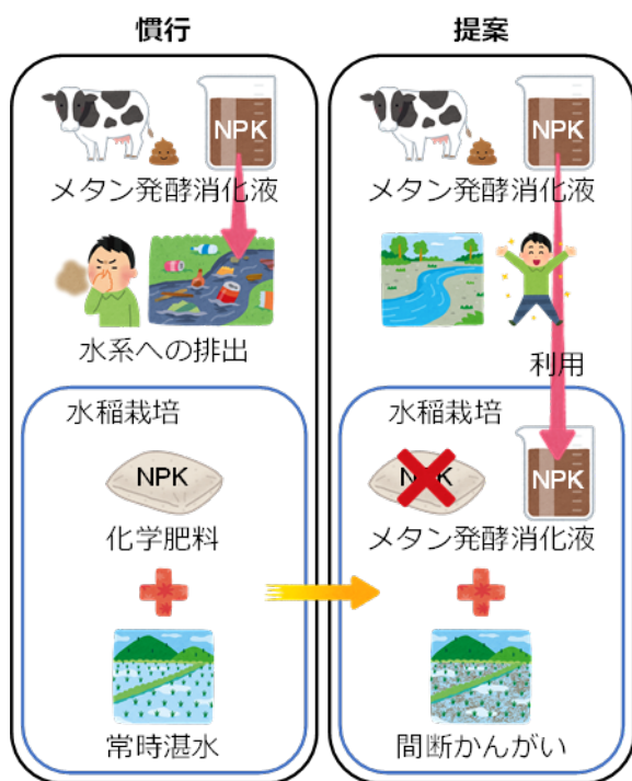
図1 未利用のメタン発酵消化液を間断かんがいと組み合わせて利用する水田からのGHG排出削減技術の提案
