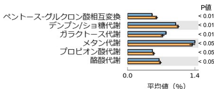
図3 CNSL給与がルーメン液中微生物群集の機能に及ぼす影響 代謝に関わる微生物群の比率を推定(オレンジ: CNSL給与あり、青: CNSL給与なし)。CNSL給与によりプロピオン酸代謝が有意に活発化することを確認。
