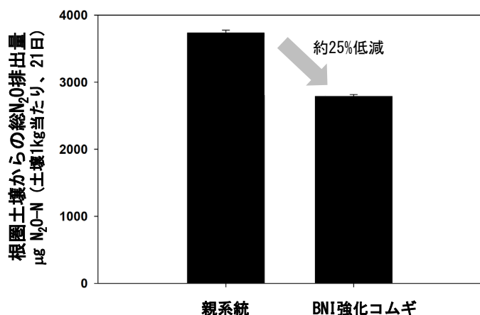
図3 BNI強化コムギと親系統の根圏土壌からの \text{N}_2\text{O} 排出量
