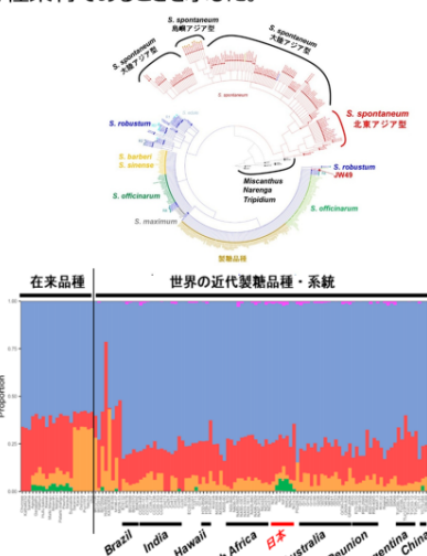
世界サトウキビ遺伝資源のミトコンドリアゲノム情報分子系統樹【上】・ 製糖品種に含まれる祖先種ゲノム割合【下】
