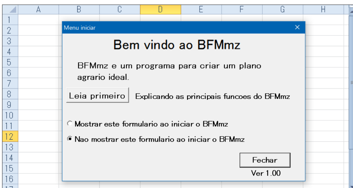
Figura 1 Menu iniciar
