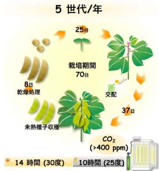
図 1 開発した技術により年 5 回のダイズの世代促進が可能になる
