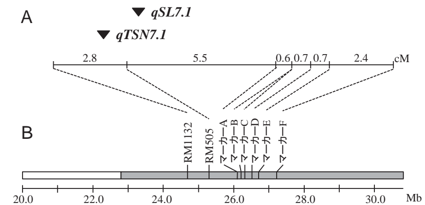
図 1 第 7 染色体長腕に検出された一穂粒数( qTSN7.1 )と粒長( qSL7.1 )の QTL の座乗位置 A:連鎖地図(▼は LOD のピーク)。B: DNA マーカーの日本晴塩基配列上での物理地図
