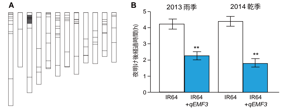
図 1 早朝開花系統(IR64+ qEMF3 )の遺伝子型模式図(A)と IR64 との開花時刻の比較(B)
