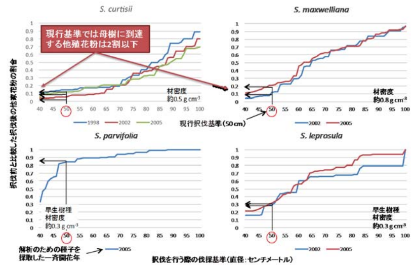
図 1. フタバガキ科林業樹種（ Shorea 属）4 樹種について択伐後の母樹に到達する他家花粉の割合を推定したシミュレーションの結果。40cm から 1cm 毎に伐採基準をスライドさせ、伐採基準以上の成木から花粉供給がない場合の他殖花粉の減少率をシミュレーション
