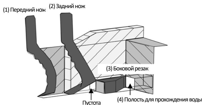
Рис. 4.3.4 Как создать кротовые дрены (функции ножей)
