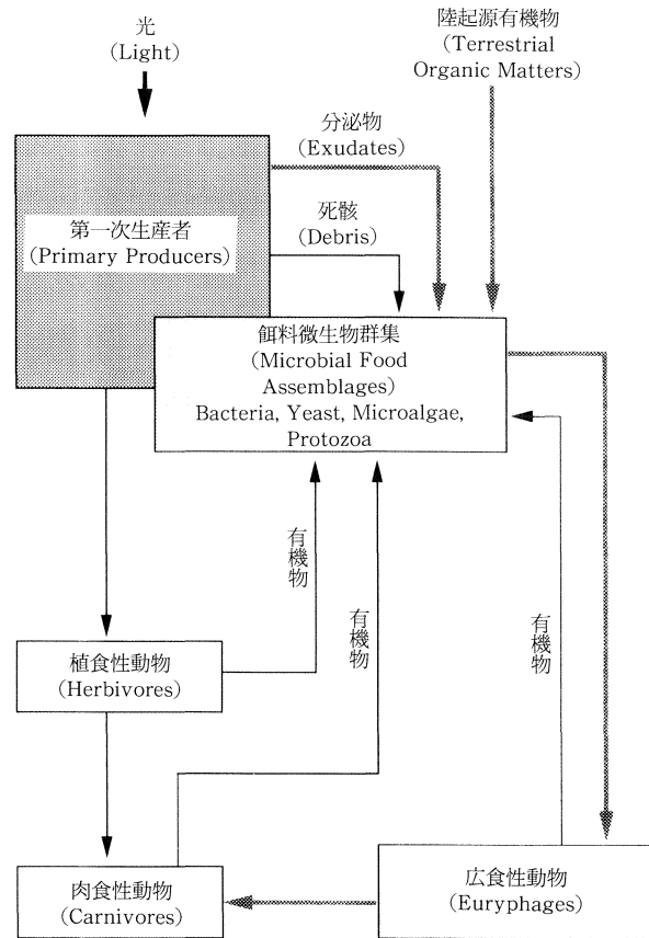
図 2 沿岸水域の食物連鎖概念図
